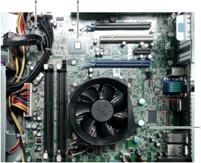
그림 2. 열 센서 및 방열판이 장착된 시스템 보드가 제거됨
